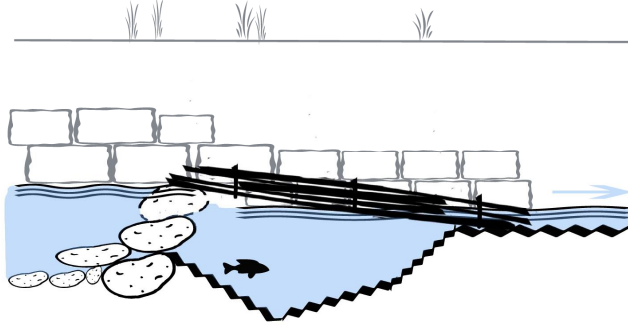
Faschine nach Schwelle Befestigung mit Ringschrauben an Blocksteinen
