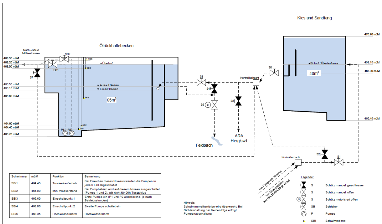
Abbildung 15: Beispiel Pumpwerk
