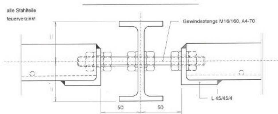
Detail Gitterbefestigung
