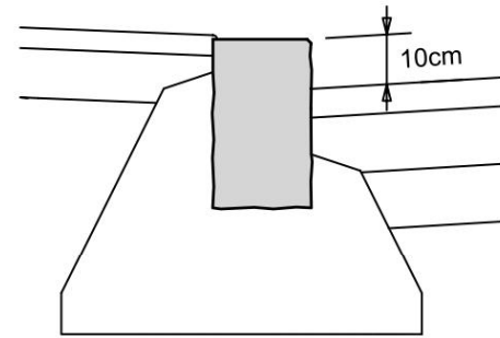
Schnitt A-A
