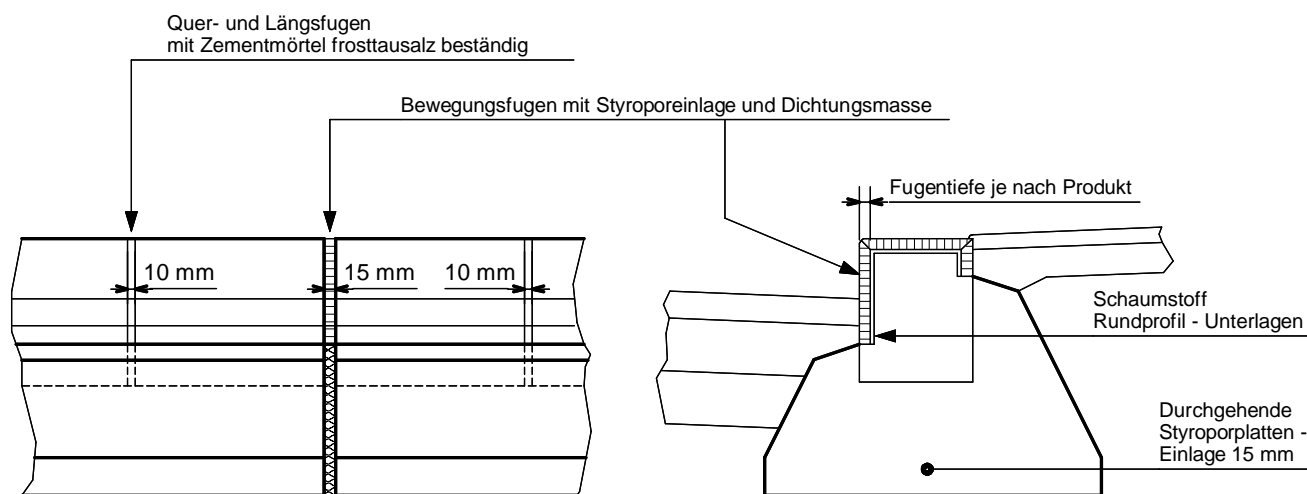
Ansicht
