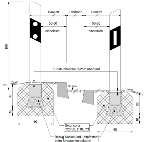
Leitpfosten freistehend
