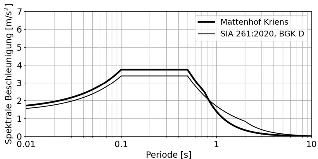
Bild 2: Elastisches Antwortspektrum für die Bemessung (fett), gültig für das Entwicklungsgebiet "Mattenhof Kriens", im Vergleich zum elastischen Antwortspektrum für die Baugrundklasse D der Norm SIA 261 (fein).
