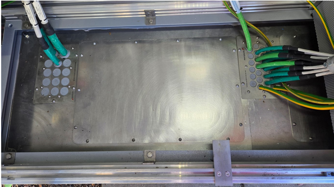
Abbildung 3: Kabinenboden mit V2A Blechboden, Cablequik-Kabeleinführungen und Revisionsöffnung
